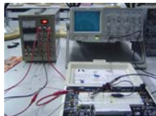
ภาพที่ 2 การสร้างวงจรออสซิลเลเตอร์แบบเวกนบริดจ์
